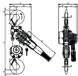
UNOplus UT-A, 6000 kg, 2 brins
