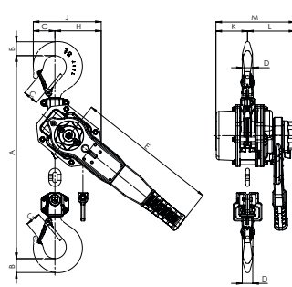
UNOplus UT-A, 3000 kg, 1 brin
