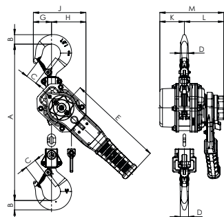
UNOplus UT-A, 1500 kg, 1 brin
